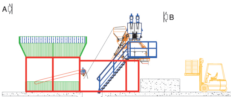
Configurazione FALCON
